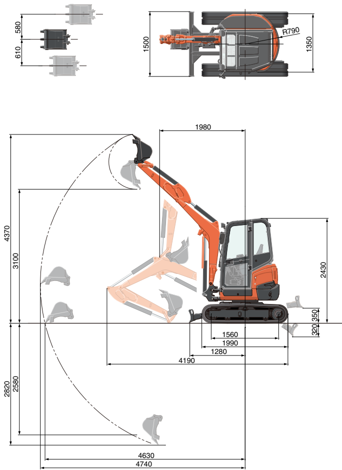
Balancín de 1300 mm Unidad: mm
